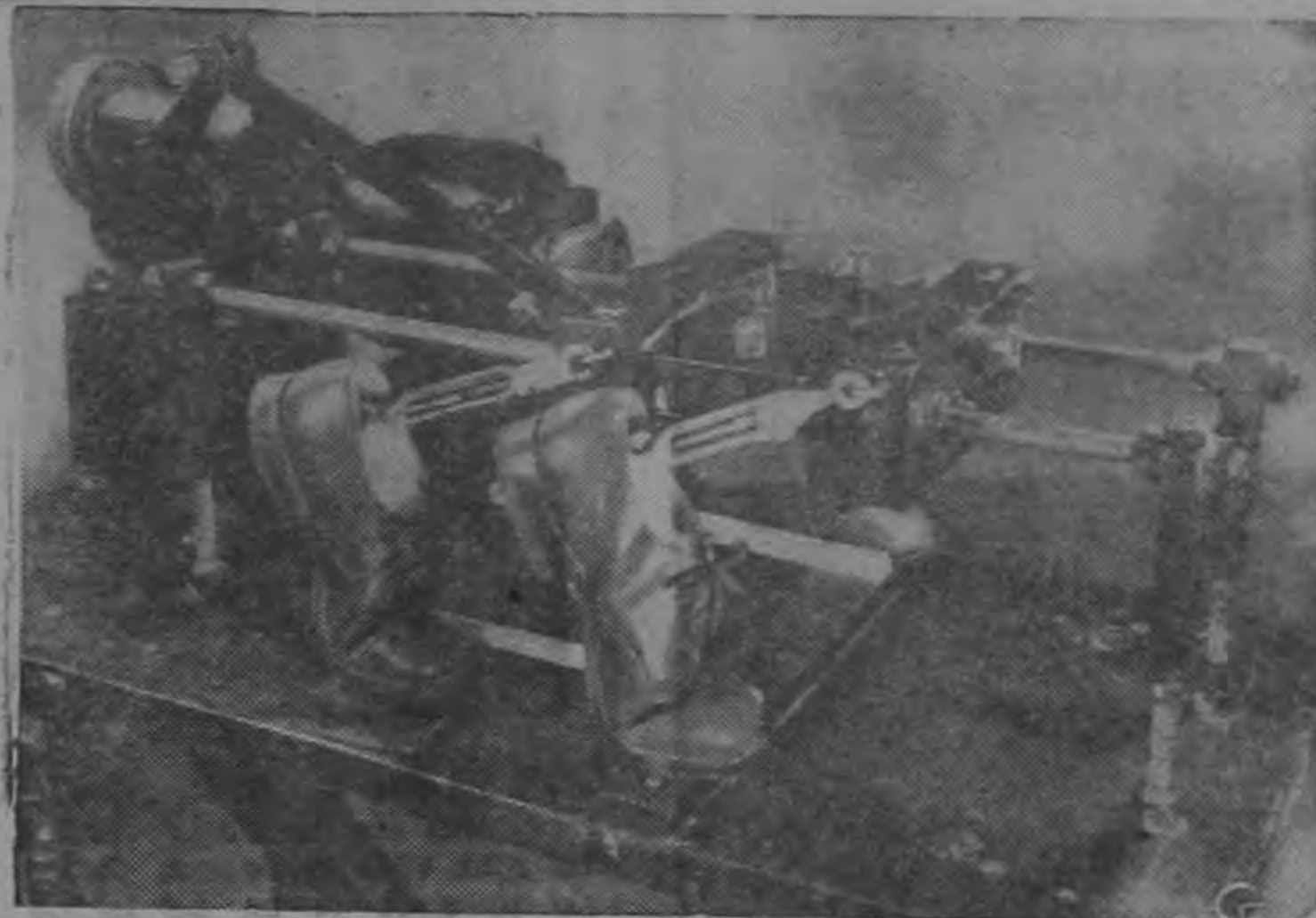
¿Se trata de un fantasma que camina? No, es que este aparato hace caminar los zapatos miles de millas para probar su duración
